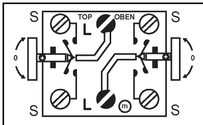
Contact aansluitingen
