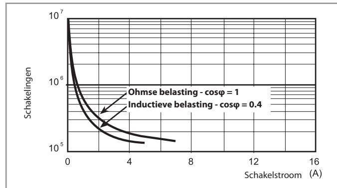
F 55 - Elektrische levensduur bij AC 4 wisselcontacten
