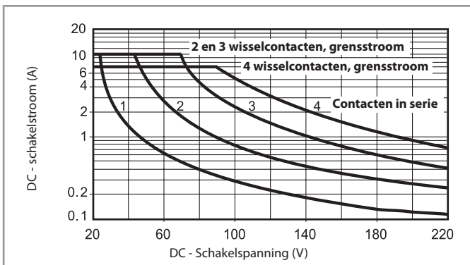
H 55 - Gelijkstroom-schakelvermogen bij DC1 - belasting
