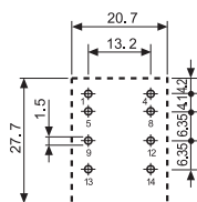
Aanzicht aansluitingen
